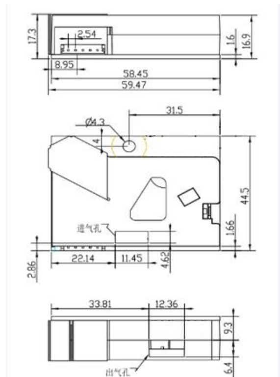
图 1: 结构尺寸图
