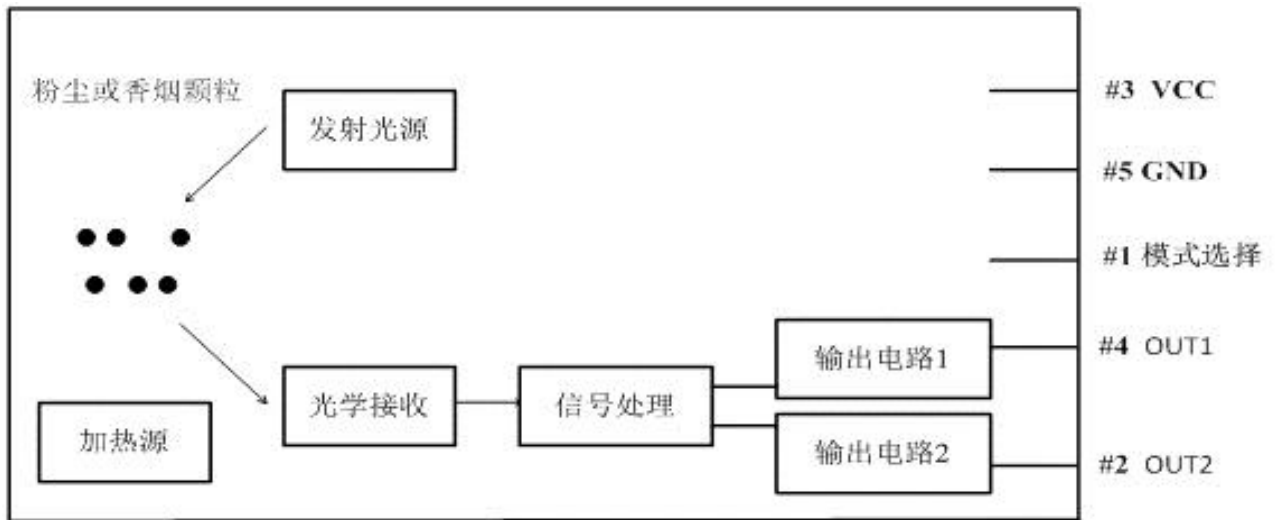
图3: 原理示意2
